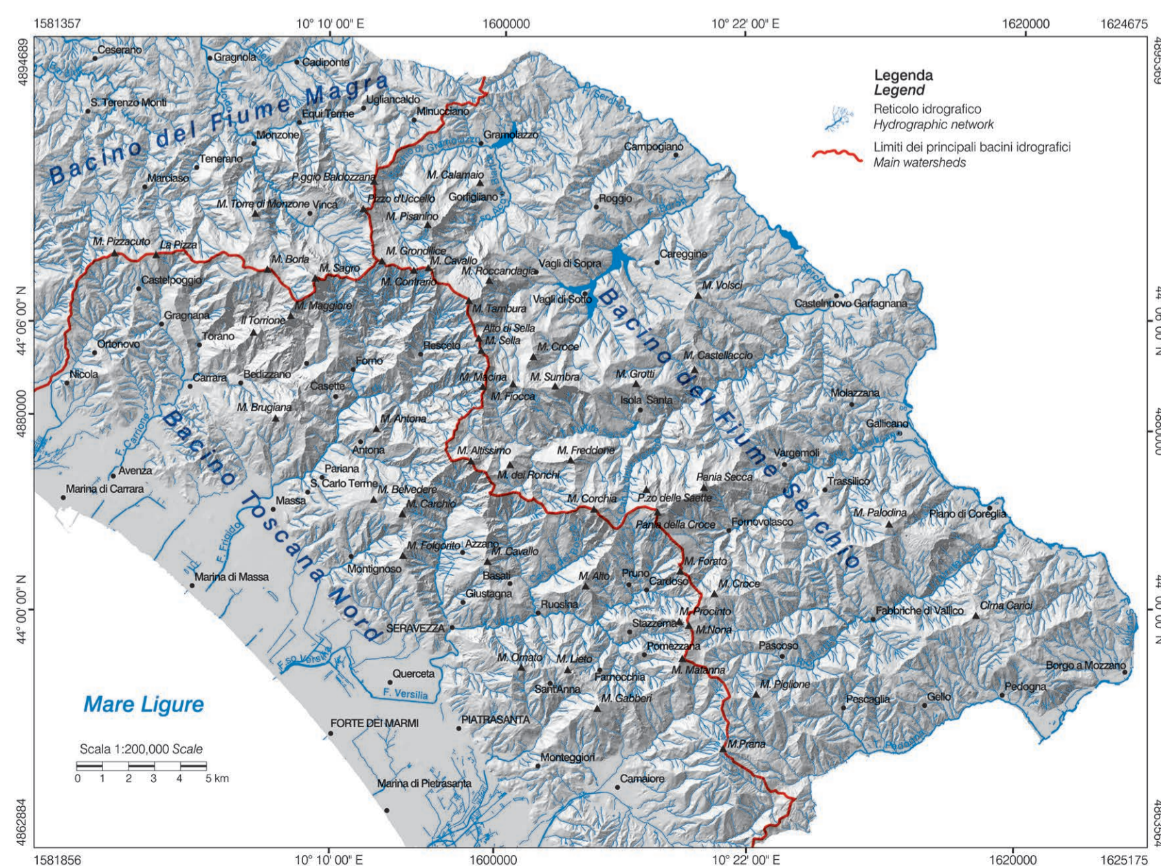
CARTA DEL RETICOLO DI DRENAGGIO DRAINAGE NETWORK MAP
