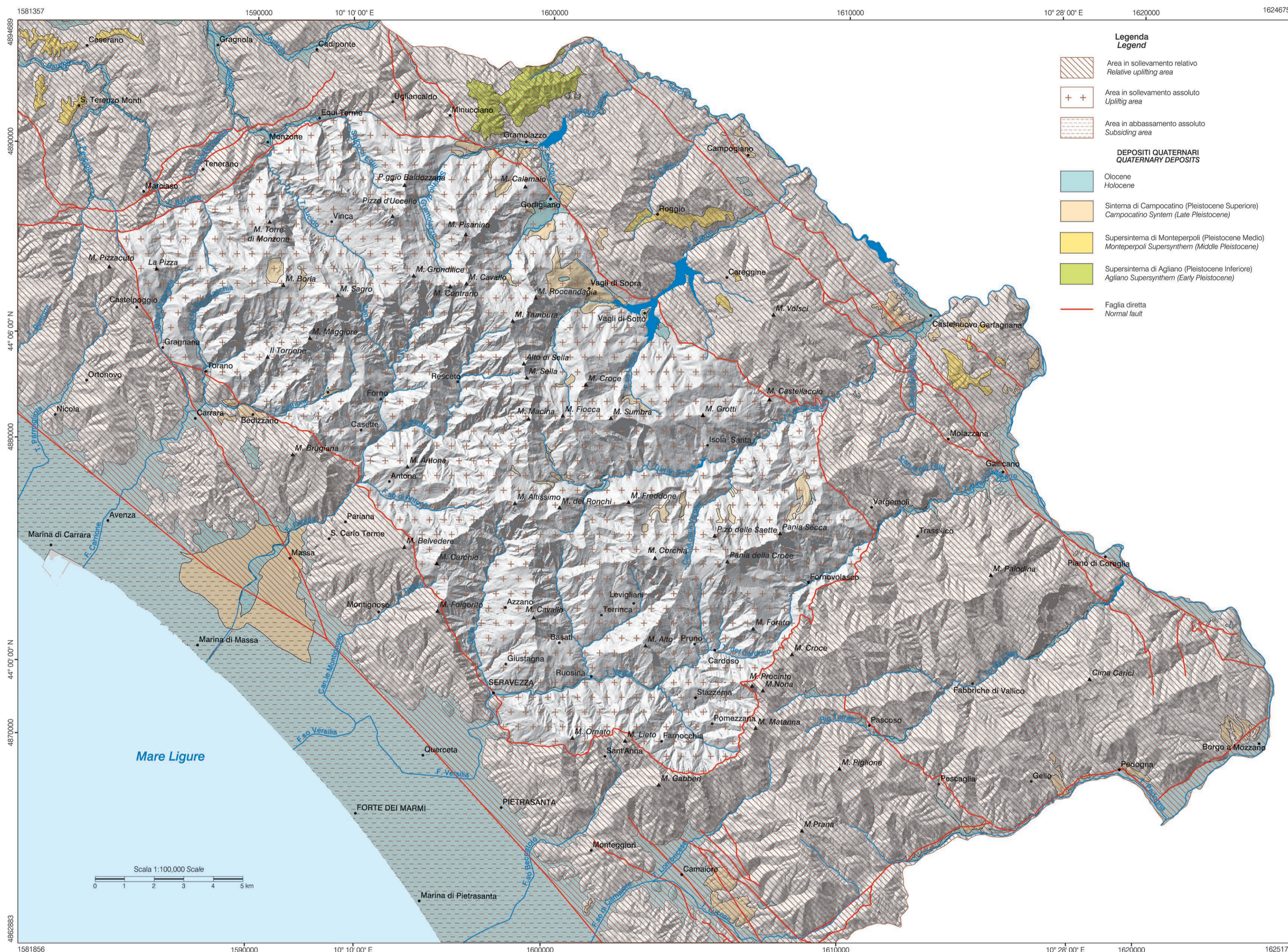
SCHEMA NEOTETTONICO NEOTECTONIC MAP
