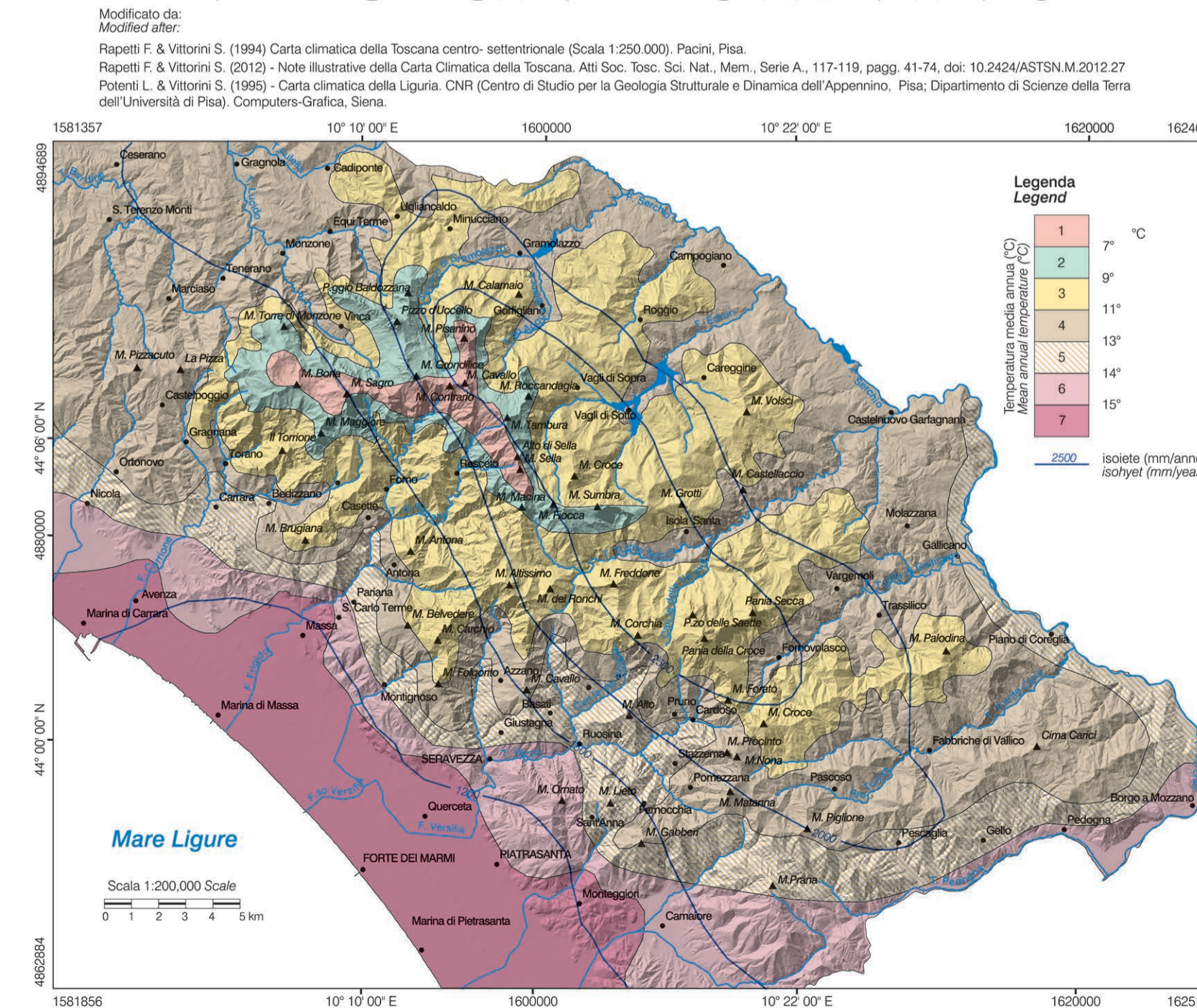
CARTA DEGLI ELEMENTI CLIMATICI MAP OF CLIMATIC ELEMENTS
