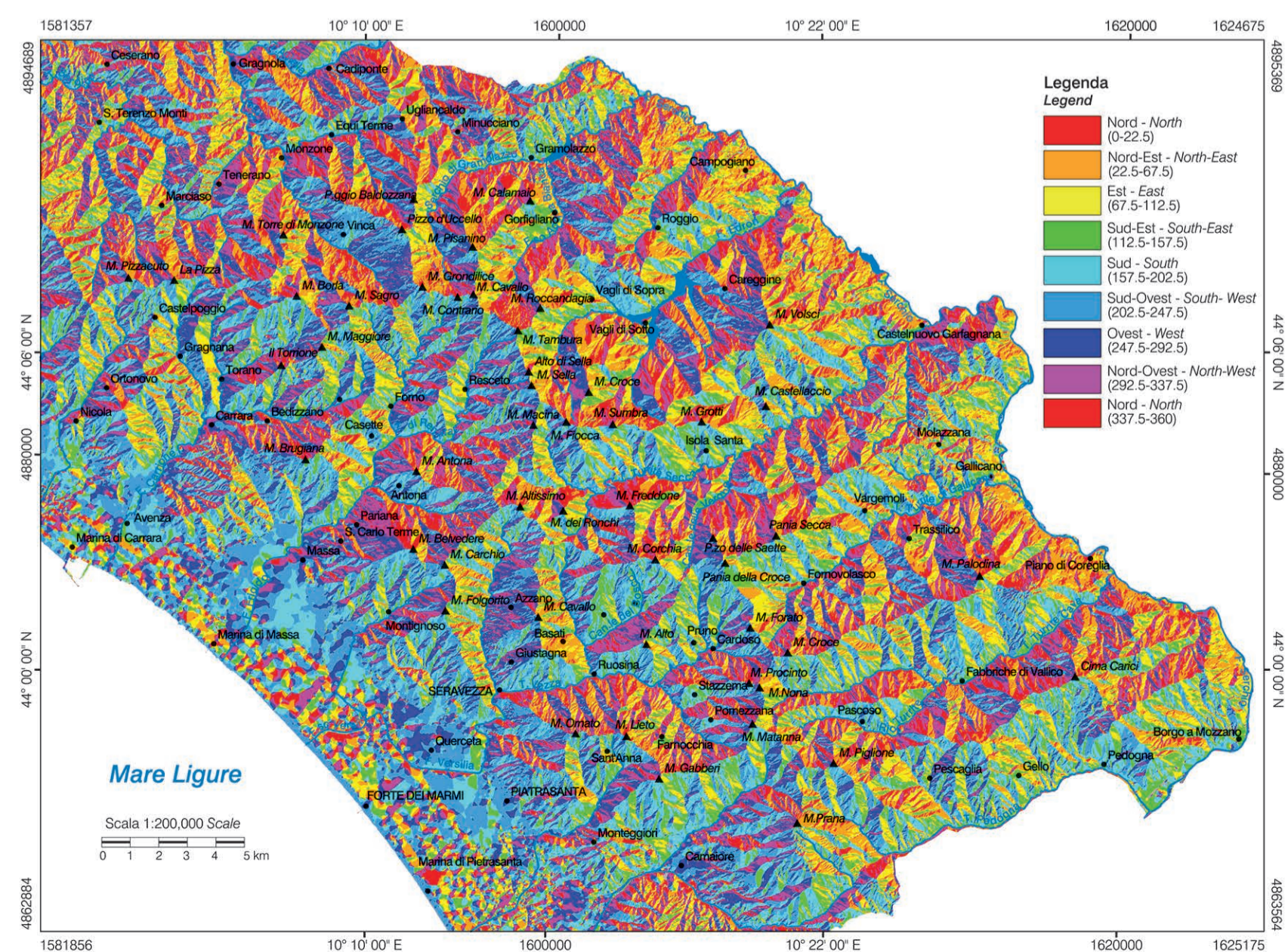
CARTA DELLE ESPOSIZIONI ASPECT MAP
